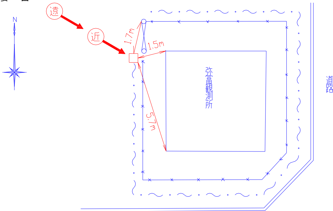
要 図
