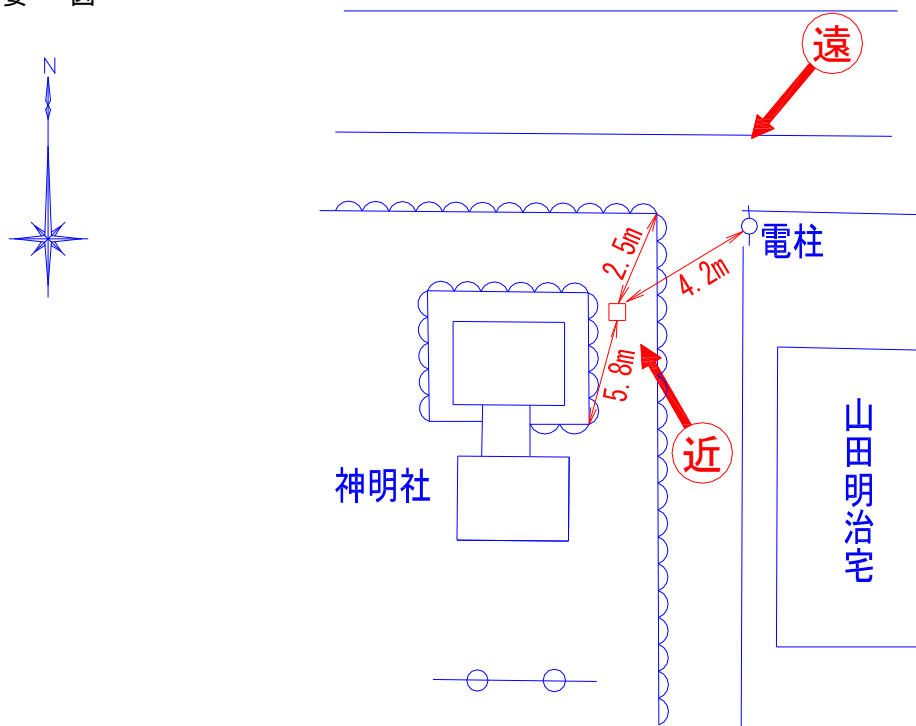
要 図
