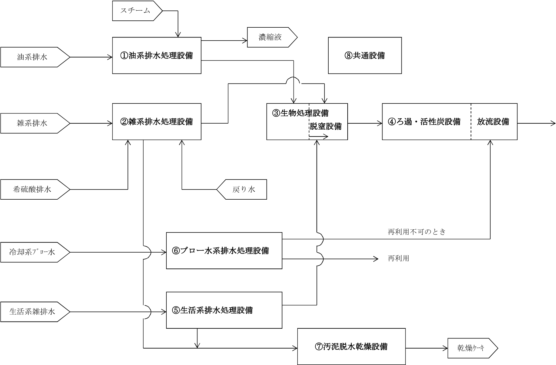
(別紙1 補足資料) 排水処理フローシート(No.2)
