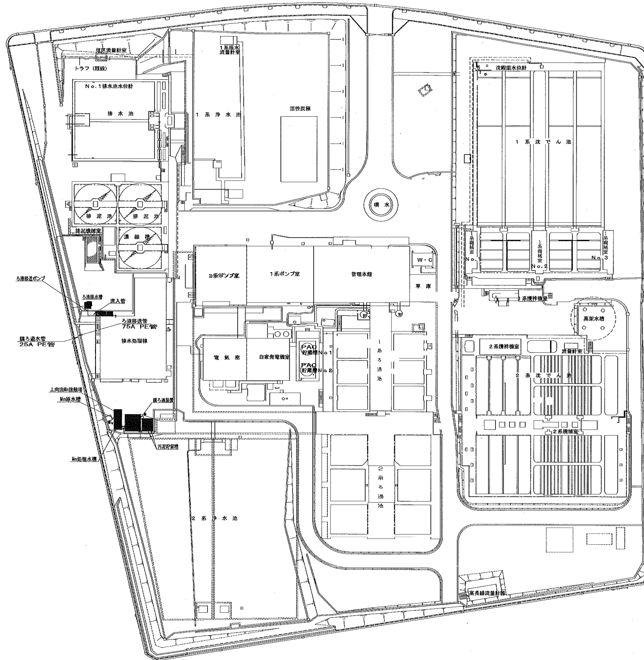
図② 高蔵寺浄水場 施設配置図
