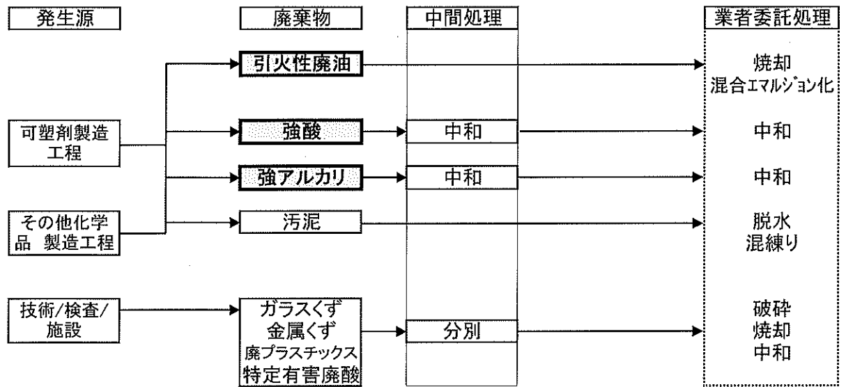
廃棄物処理フローシート(産業廃棄物)
