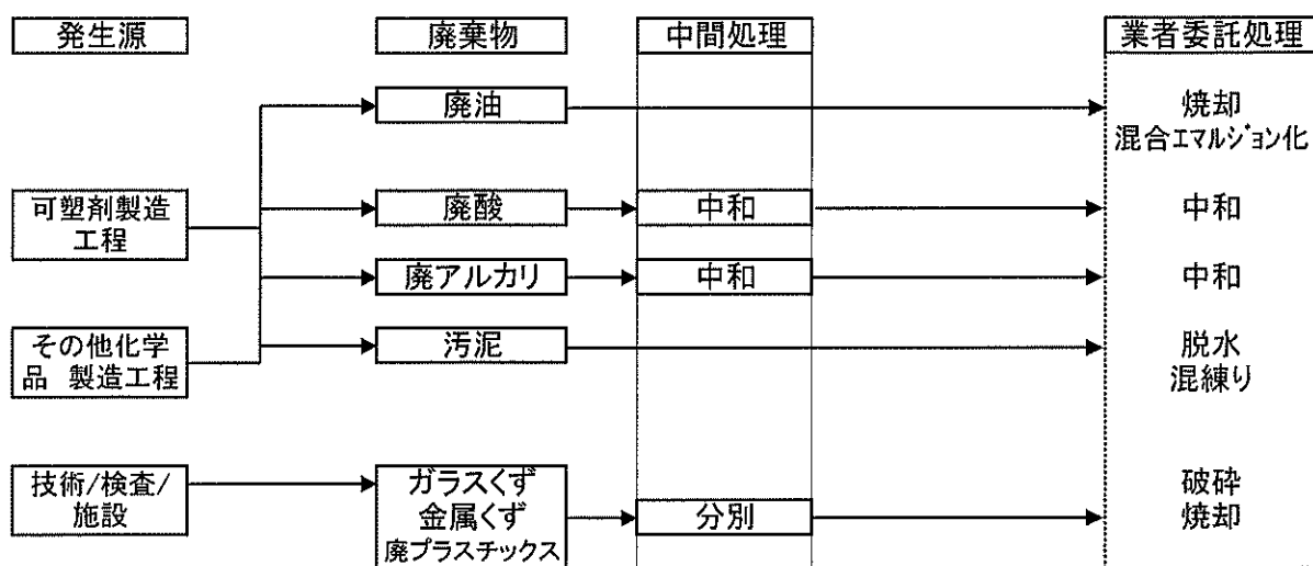
廃棄物処理フローシート(産業廃棄物)
