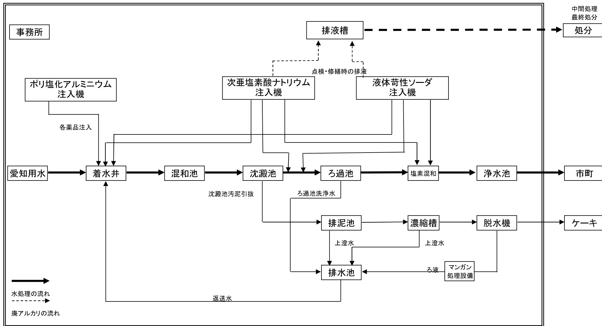
図③ 高蔵寺浄水場 廃アルカリ処理のフローシート
