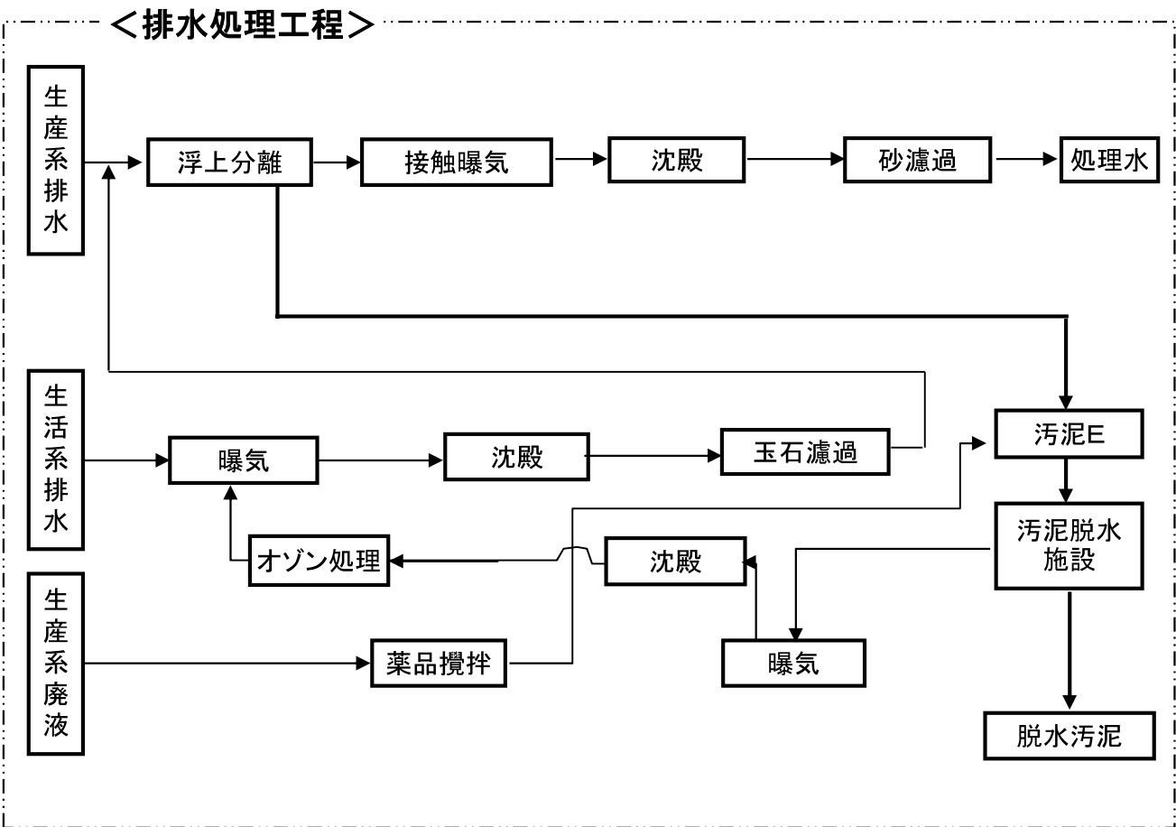
図2 排水処理フローシート
