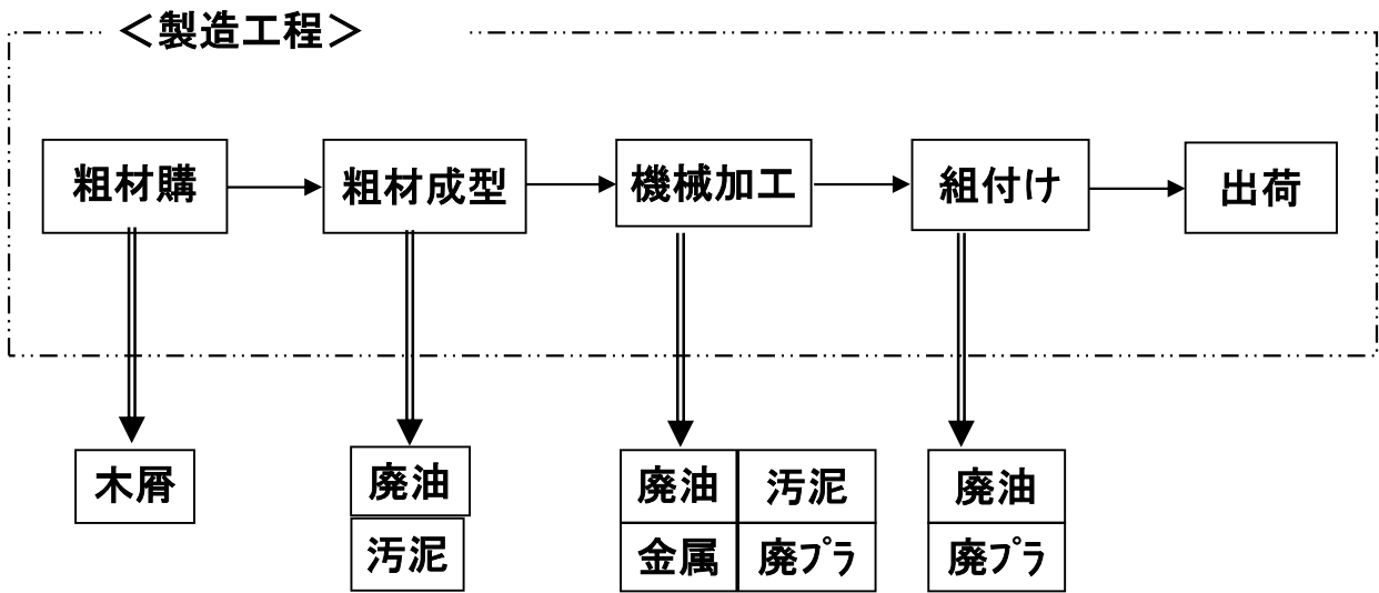
図1 自動車部品製造工程及び産業廃棄物発生工程フローシート
