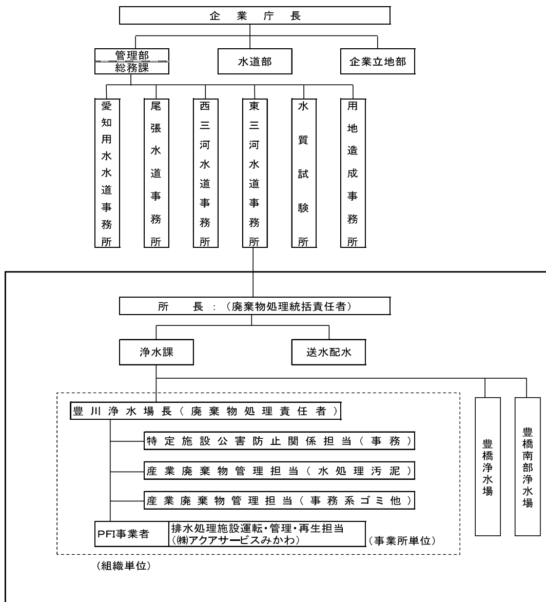
豊川浄水場 廃棄物管理組織図
