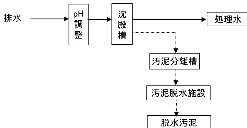
別図3 排水処理 フローシート
