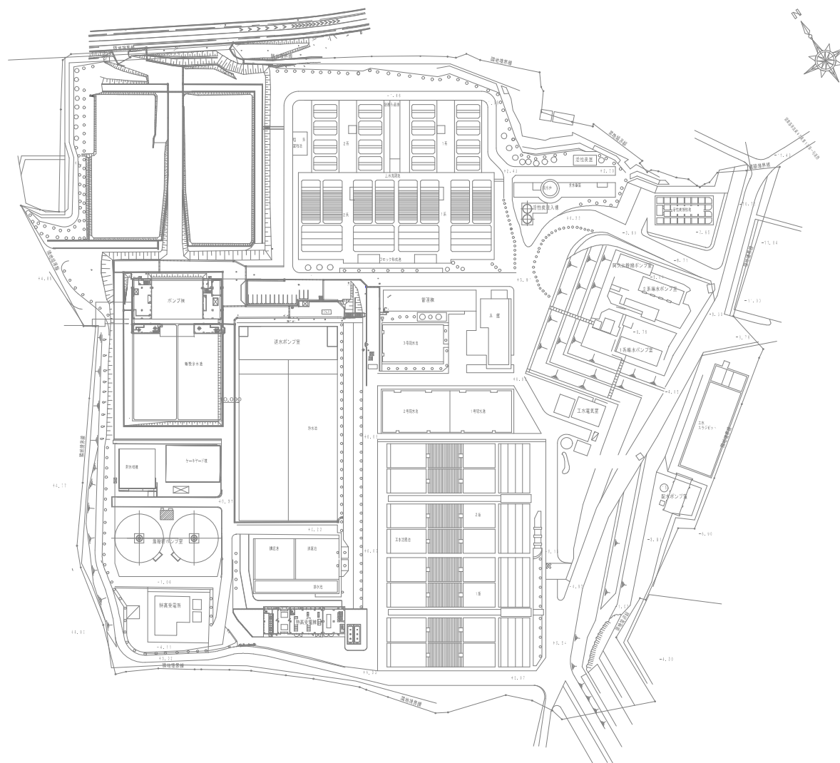
一般平面図 1/1,000
