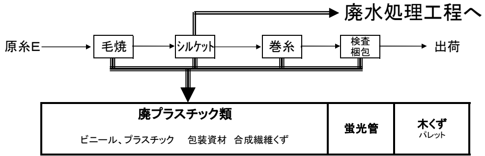
図4 連シル糸製造部門フローシート
