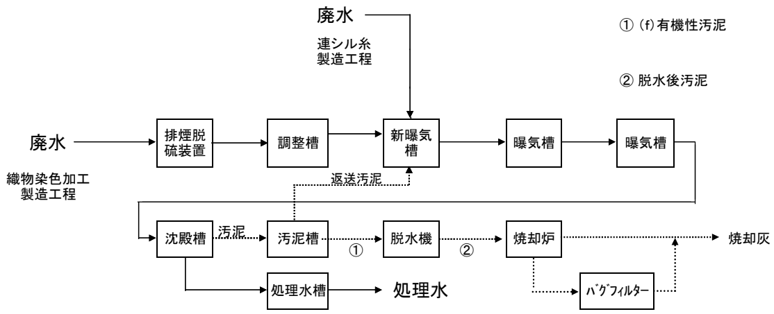
図5 廃水処理工程フローシート
