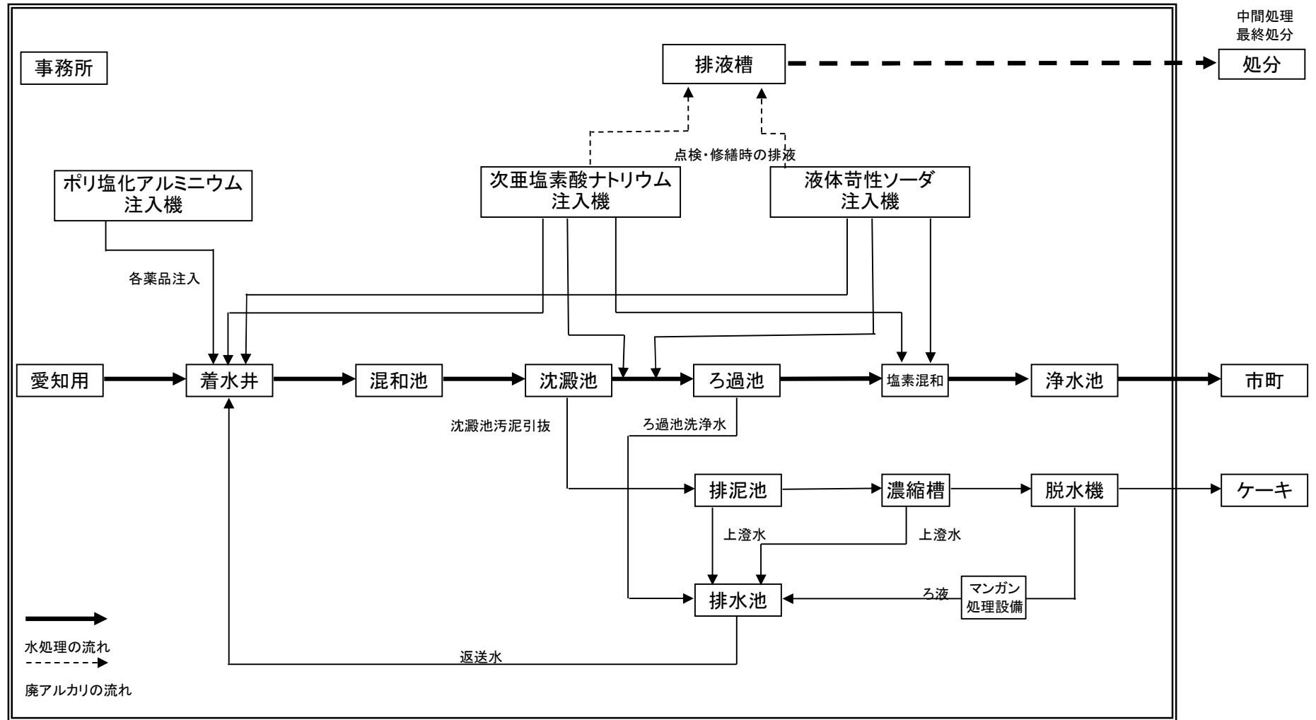
図④ 高蔵寺浄水場 廃アルカリ処理のフローシート
