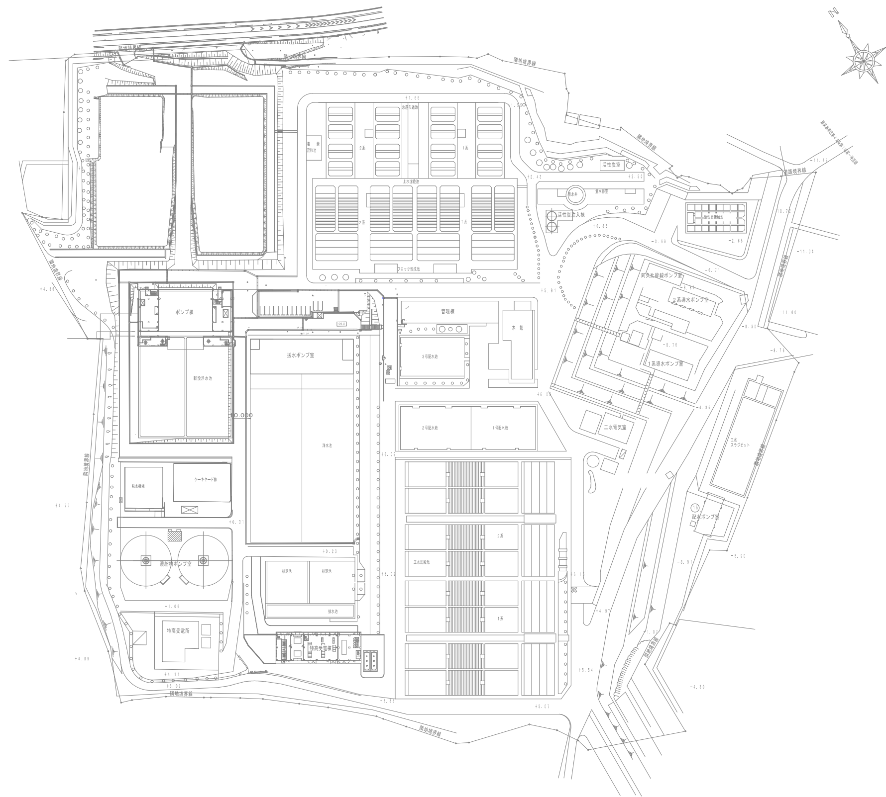
一般平面図 1/1,000
