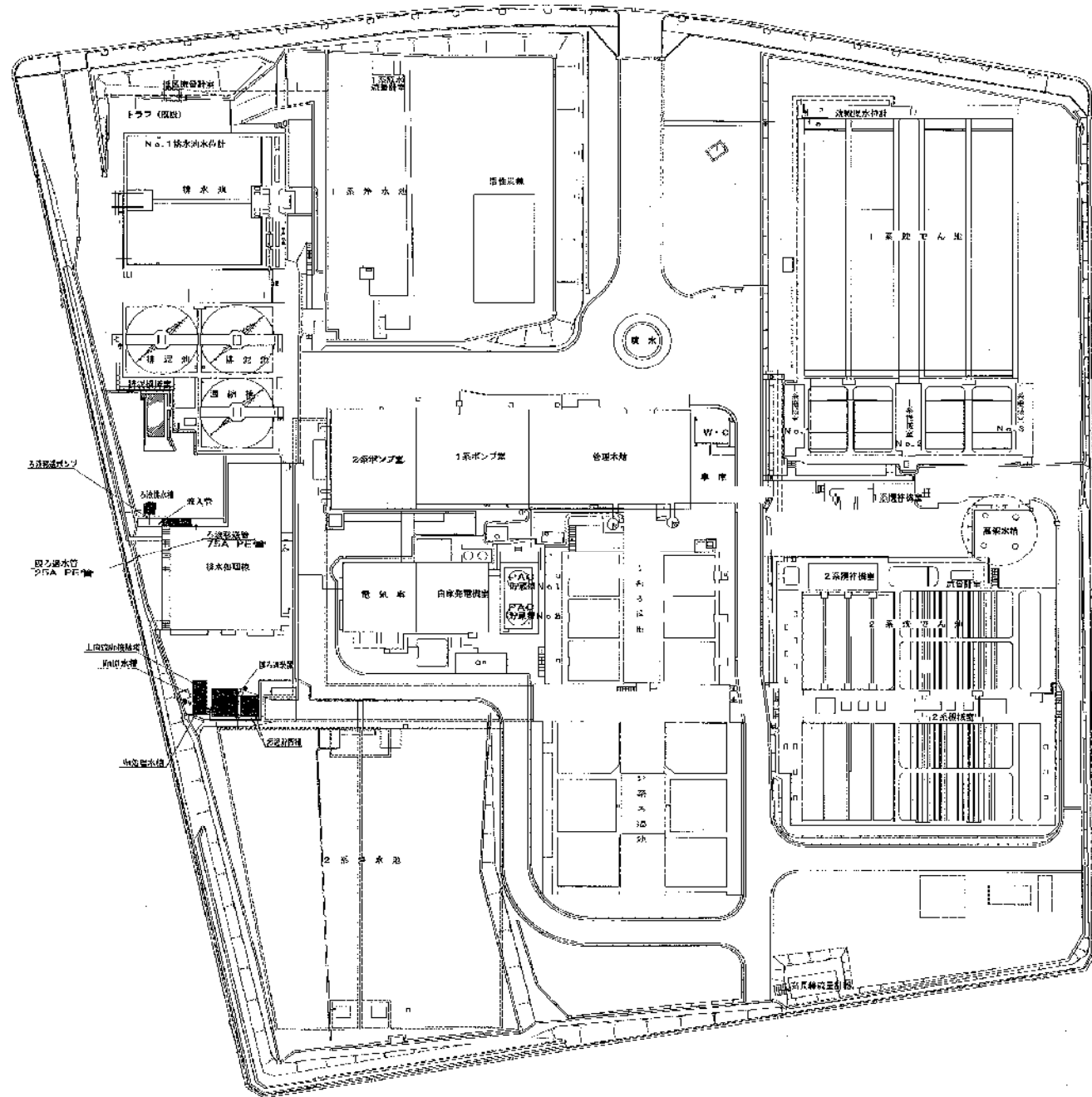
図② 高蔵寺浄水場 施設配置図
