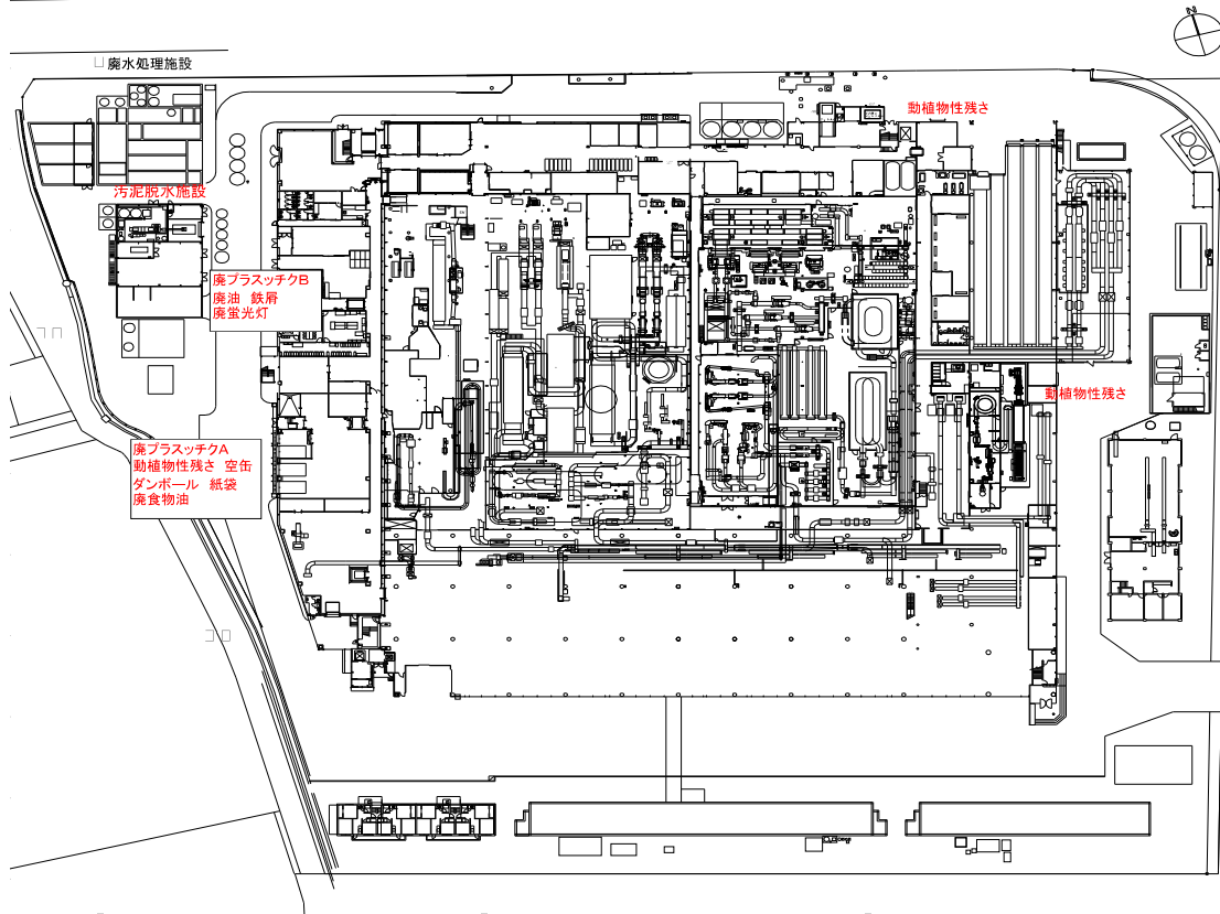
犬山工場 1階配置図
