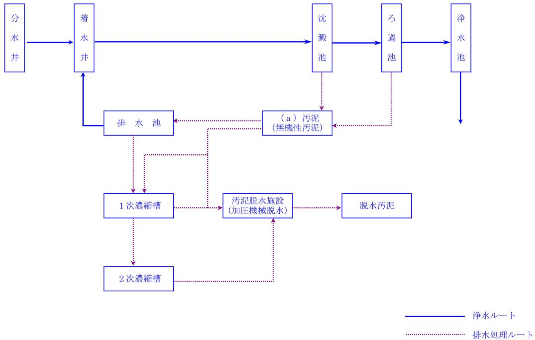
図 3 排水処理フローシート
