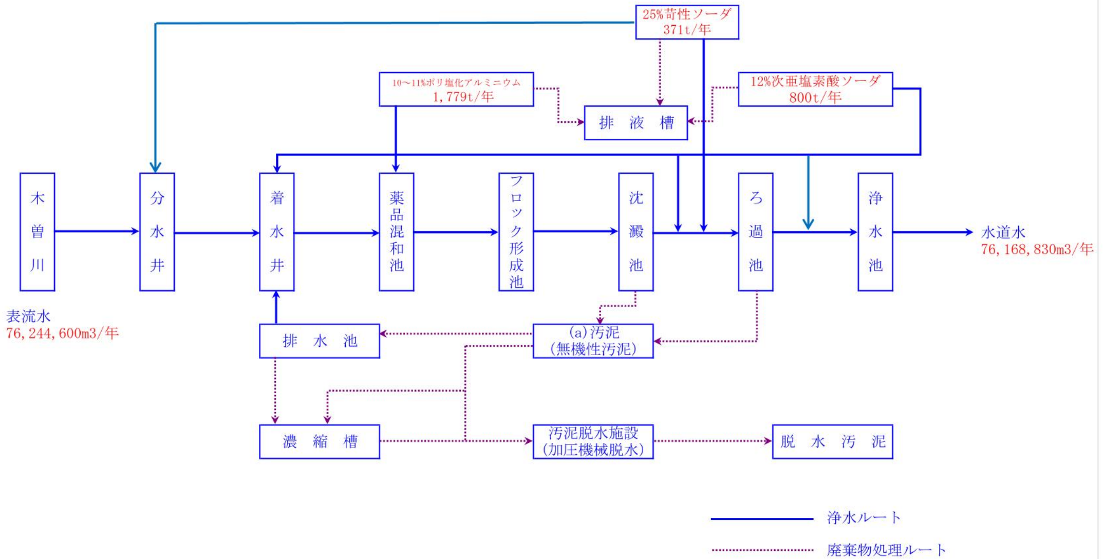
図 2 水道水製造フローシート
