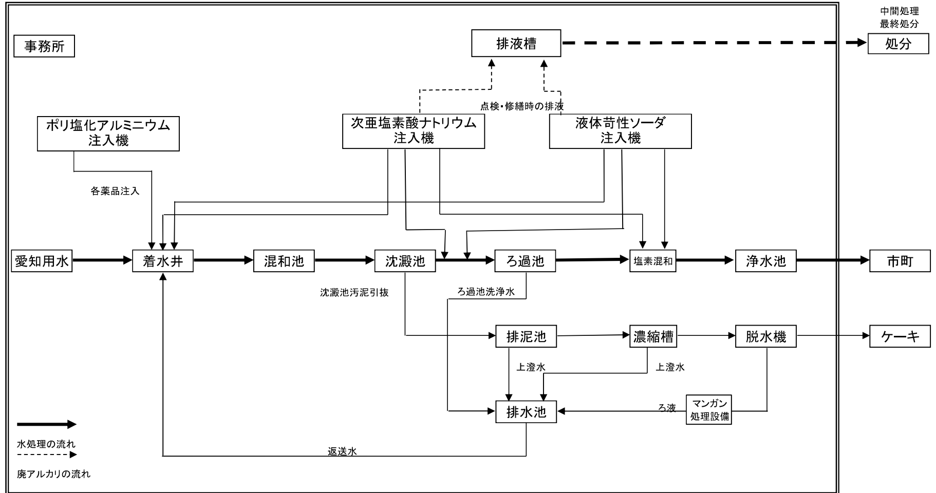
図③ 高蔵寺浄水場 廃アルカリ処理のフローシート
