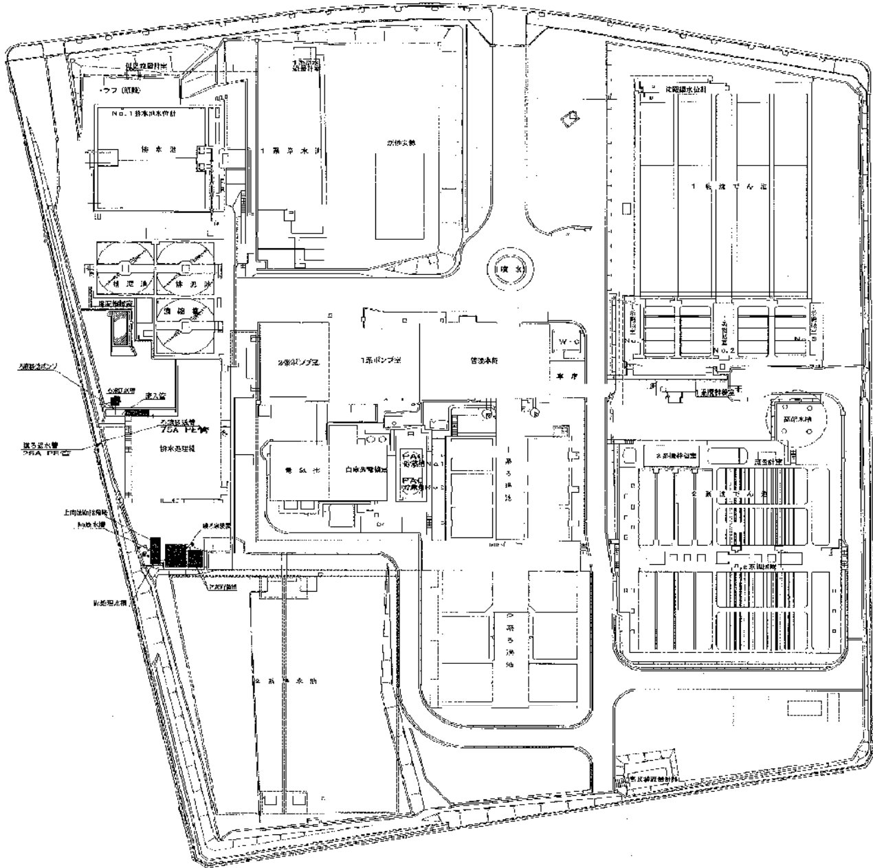
図② 高蔵寺浄水場 施設配置図
