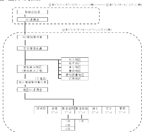
(管理体制図)
