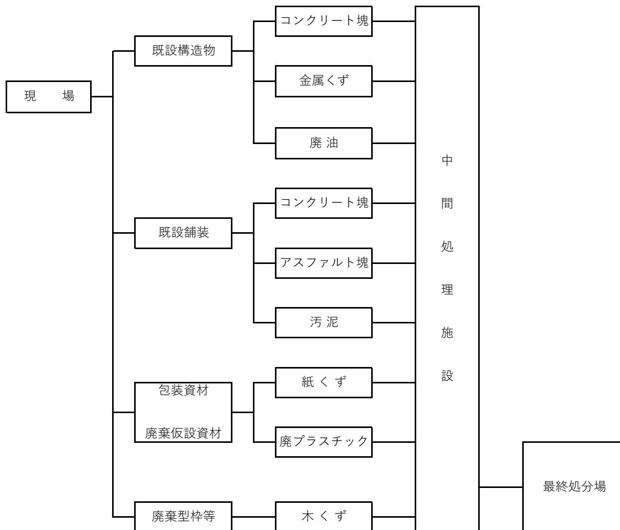
産業廃棄物発生フロー図
