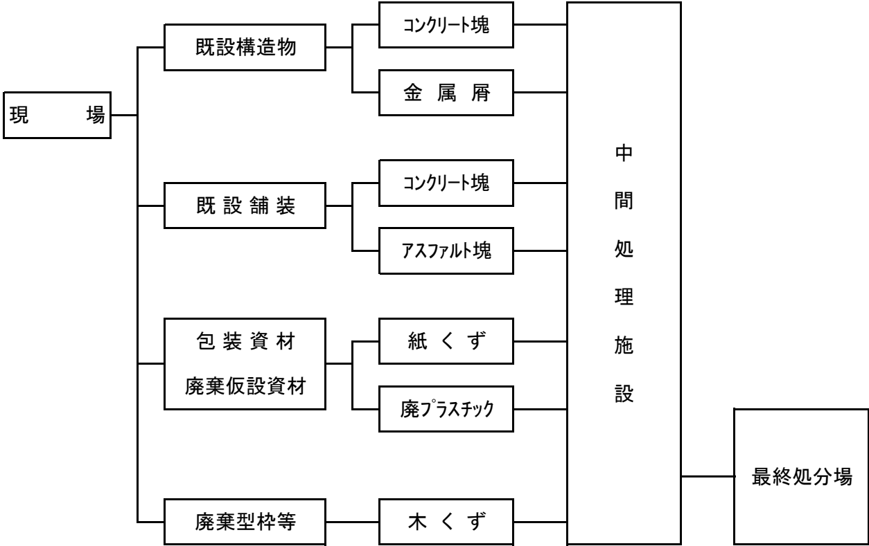
産業廃棄物発生フロー図
