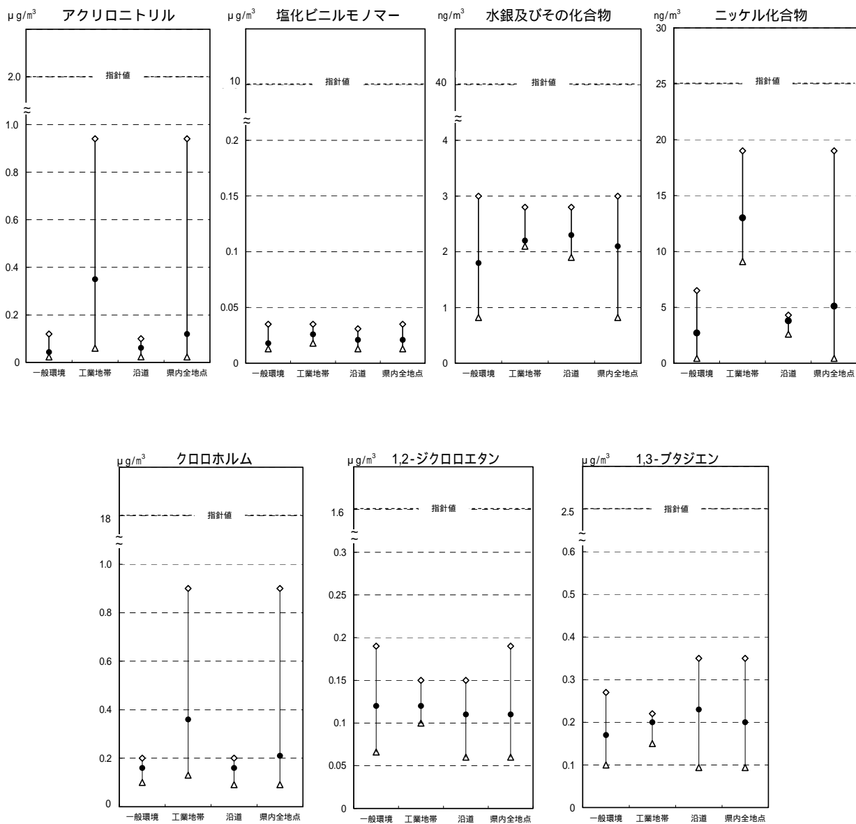
図 4 - 2 - 3 平成19年度における指針値の定められている物質の調査結果
