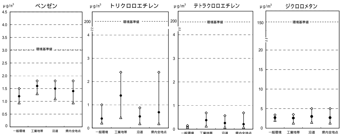
図4 - 2 - 2 平成19年度における環境基準の定められている物質の調査結果 ( : 平均値 : 最大値 : 最小値 )
