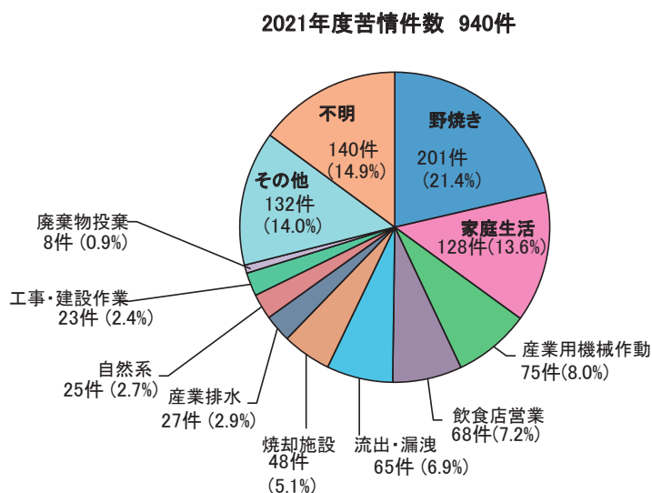
図4-3-1 悪臭に係る発生源別苦情件数
