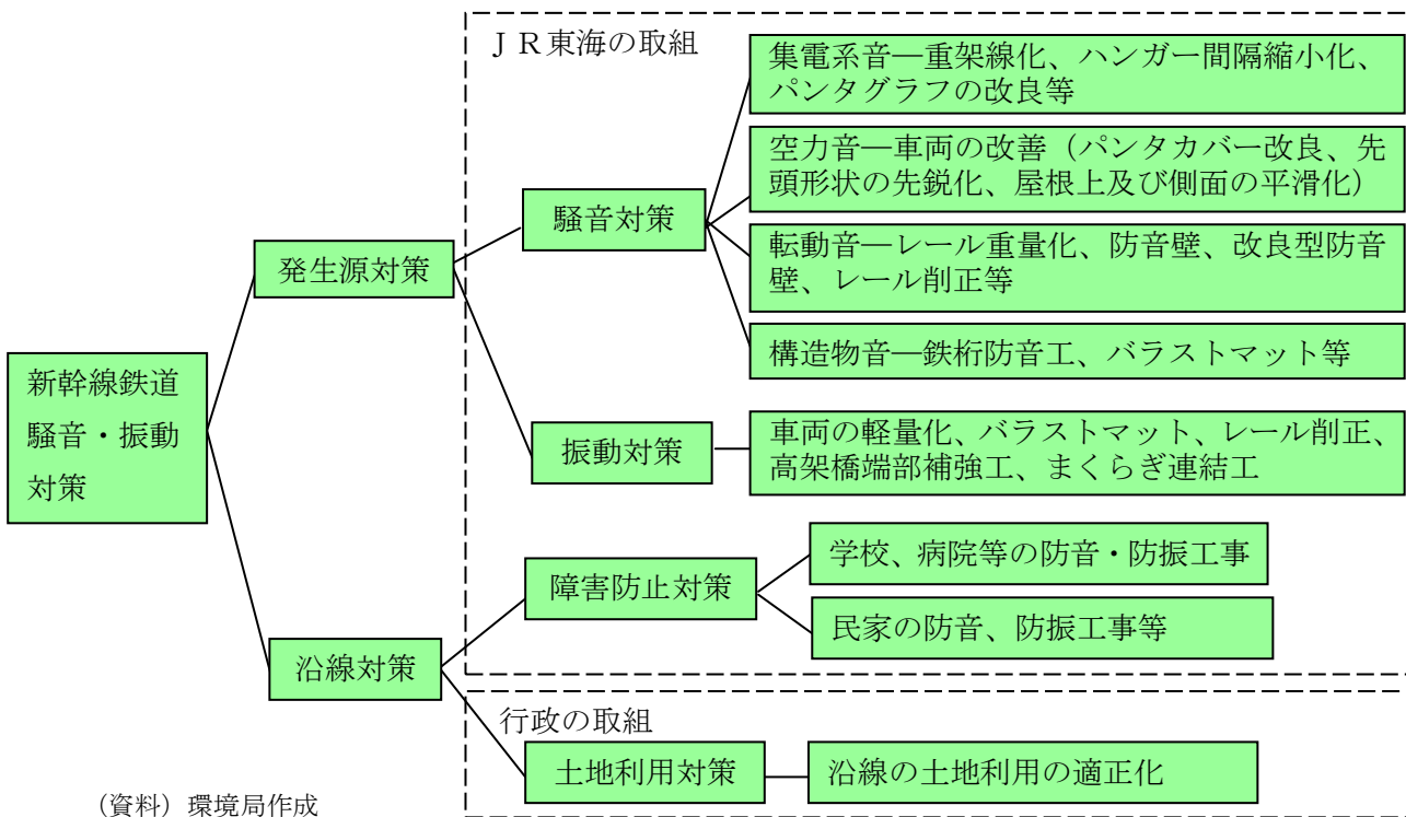
図 3-3-2 新幹線鉄道騒音・振動対策の体系
