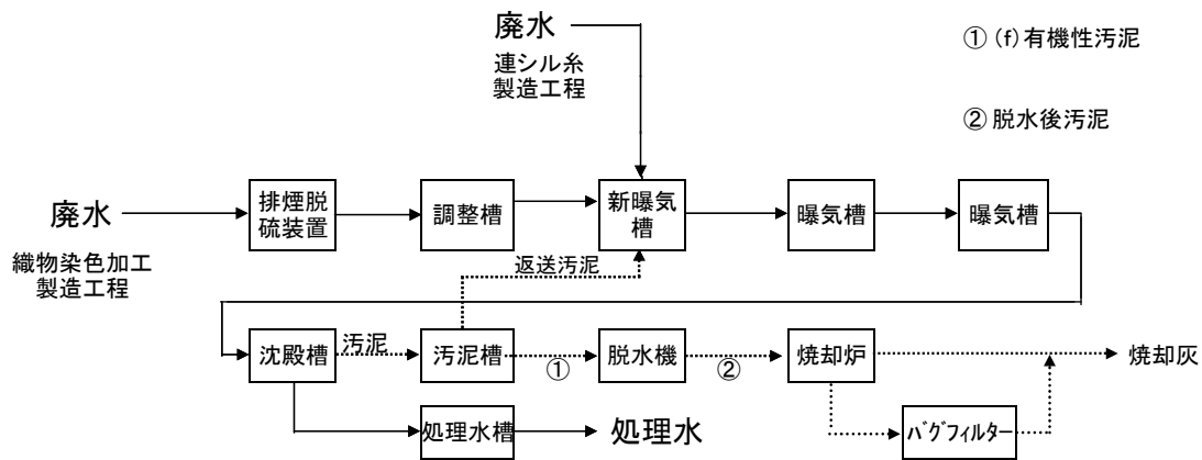
図5 廃水処理工程フローシート
