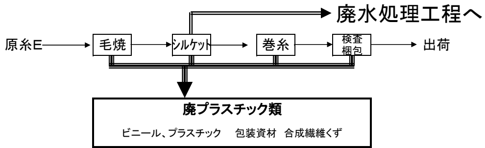
図4 連シル糸製造部門フローシート
