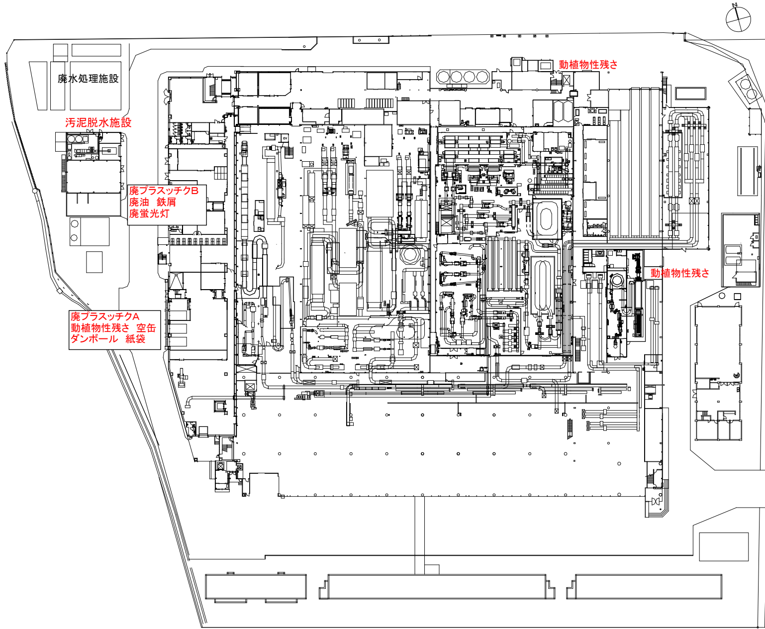
犬山工場 1階配置図
