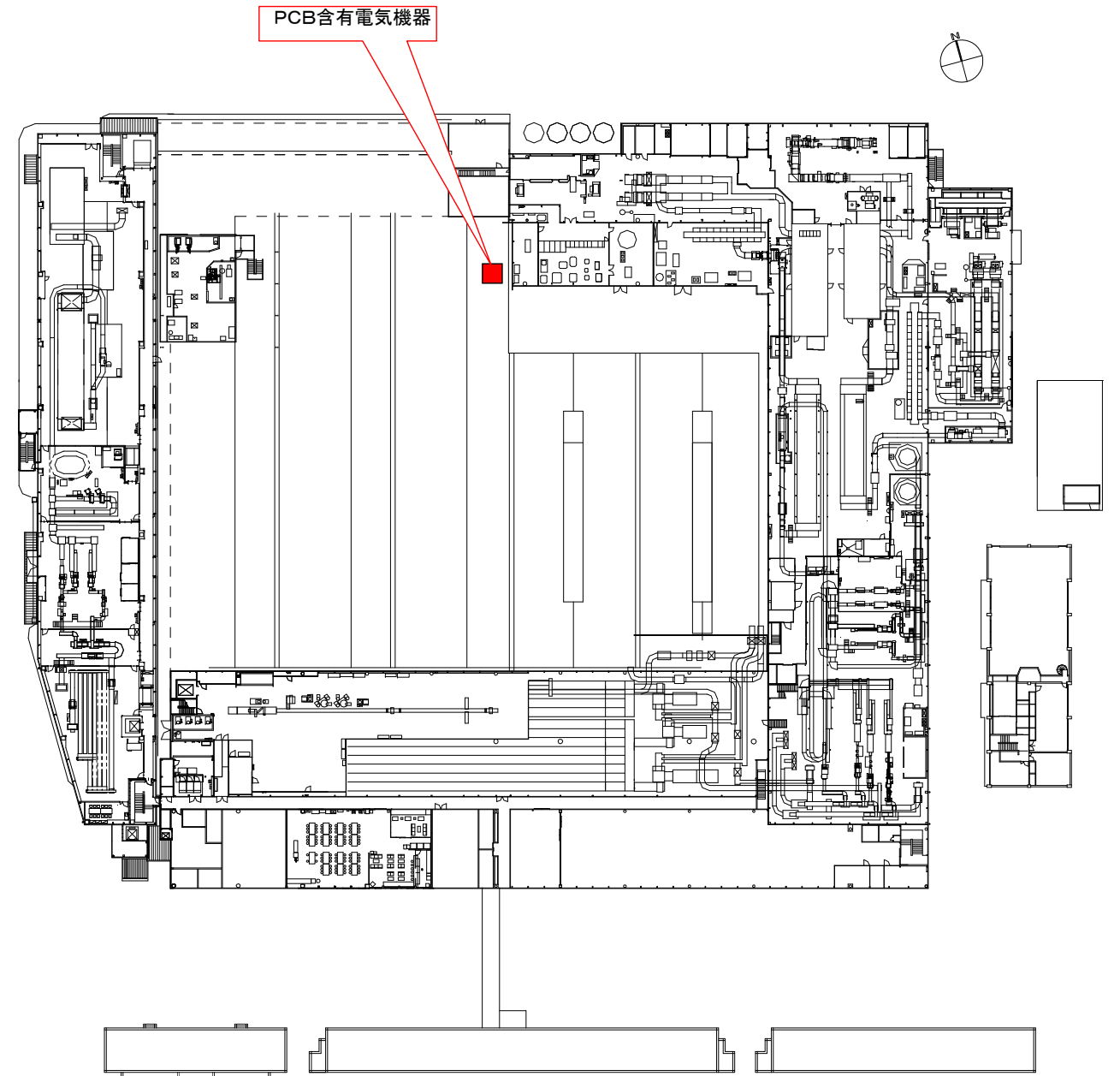
犬山工場 2階配置図
