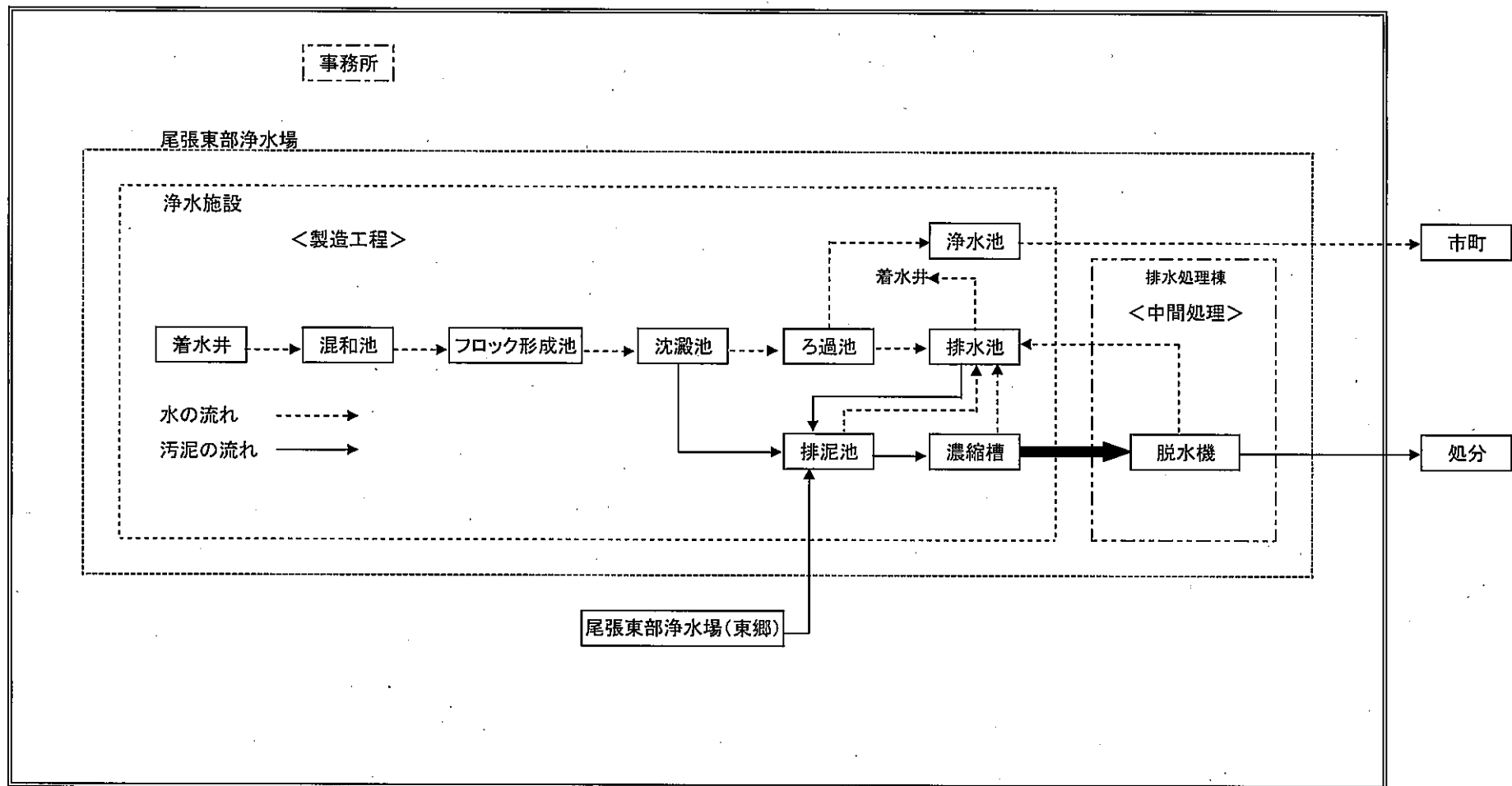
図④ 尾張東部浄水場 汚泥処理のフローシート
