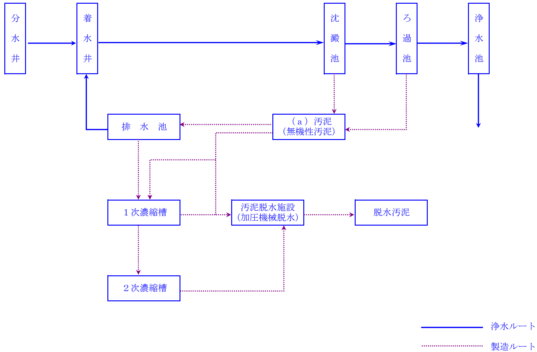
図 3 排水処理フローシート
