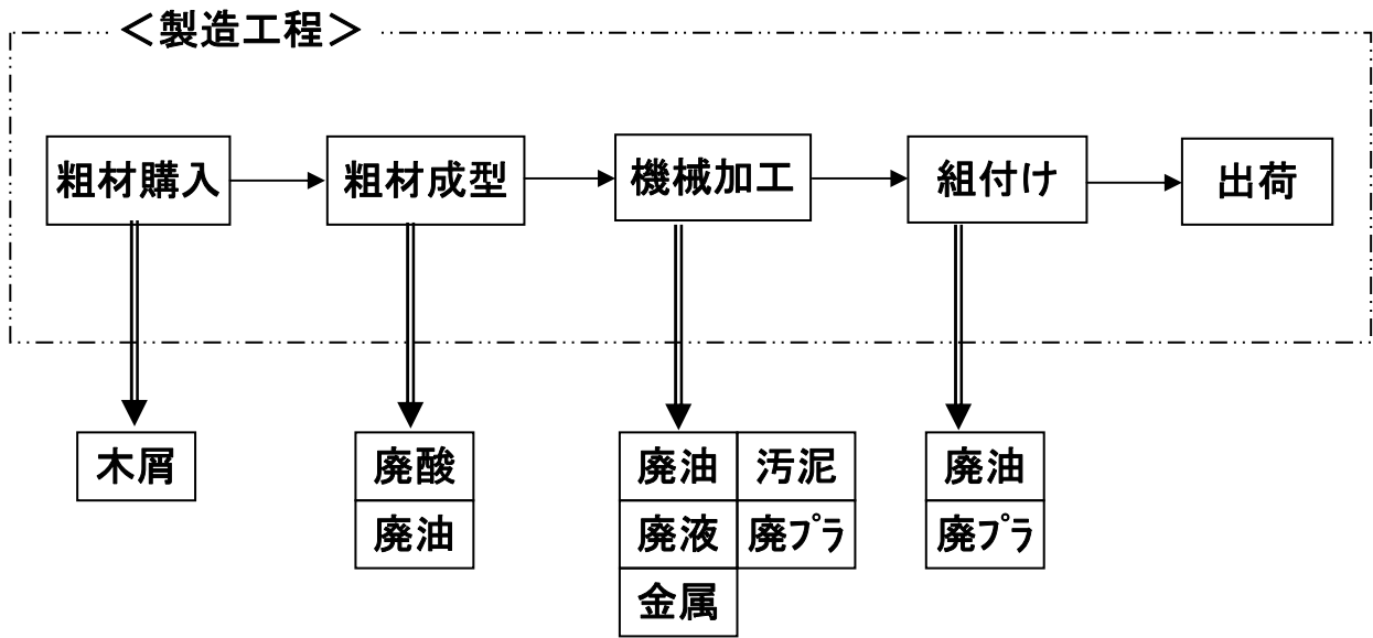
図1 自動車部品製造工程及び産業廃棄物発生工程フローシート
