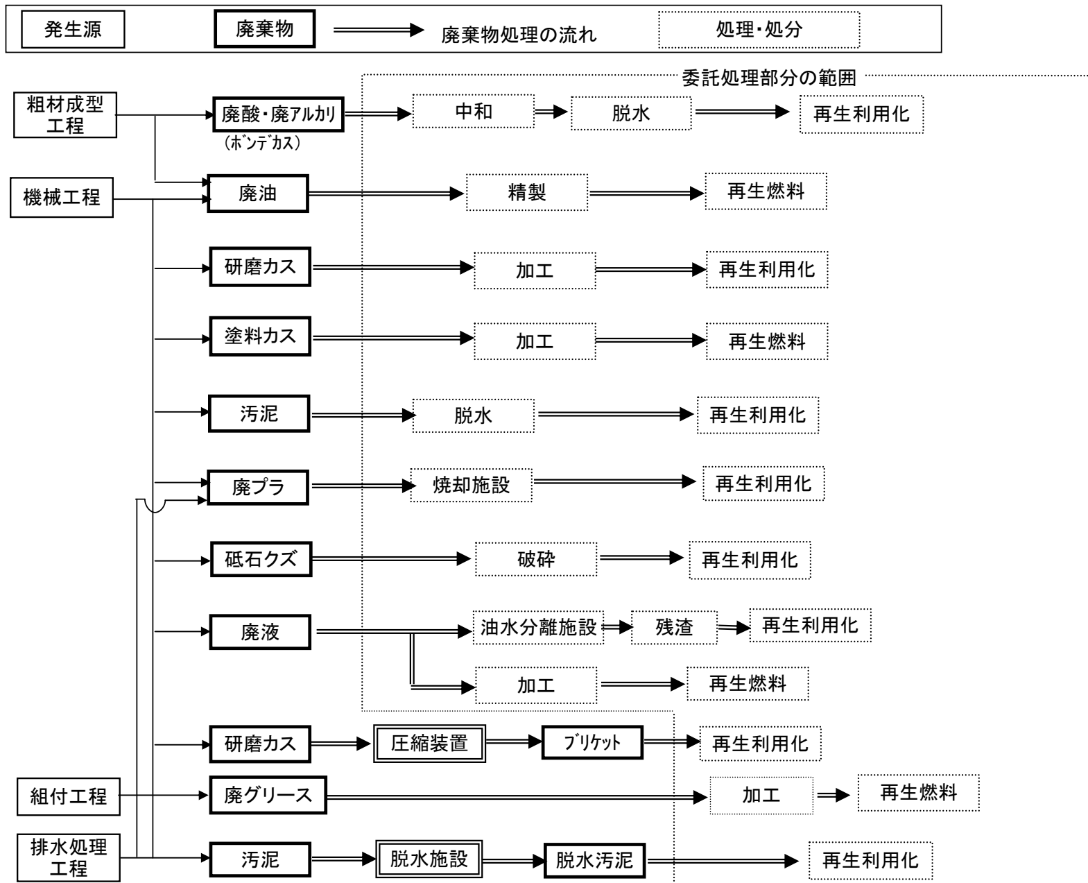
図3 廃棄物処理フロー図(産業廃棄物)
