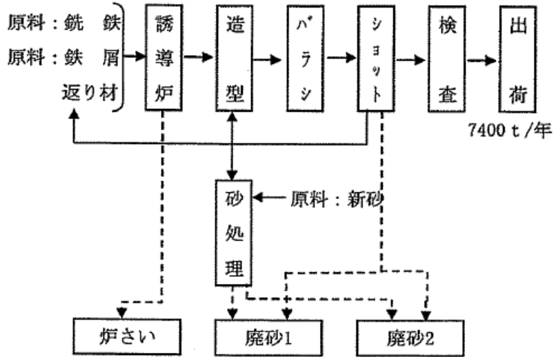
(エ) 製造工程フロー (図1)
