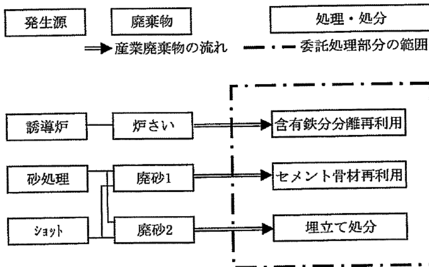
(ロ) 廃棄物処理フロー現状 (図3)
