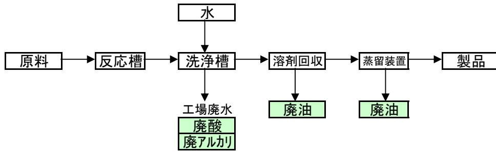
可塑剤製造フローシート
