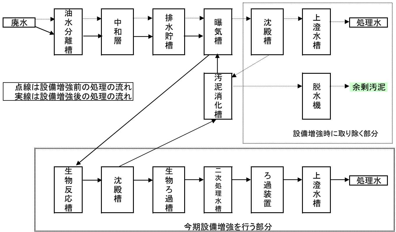
排水処理フローシート
