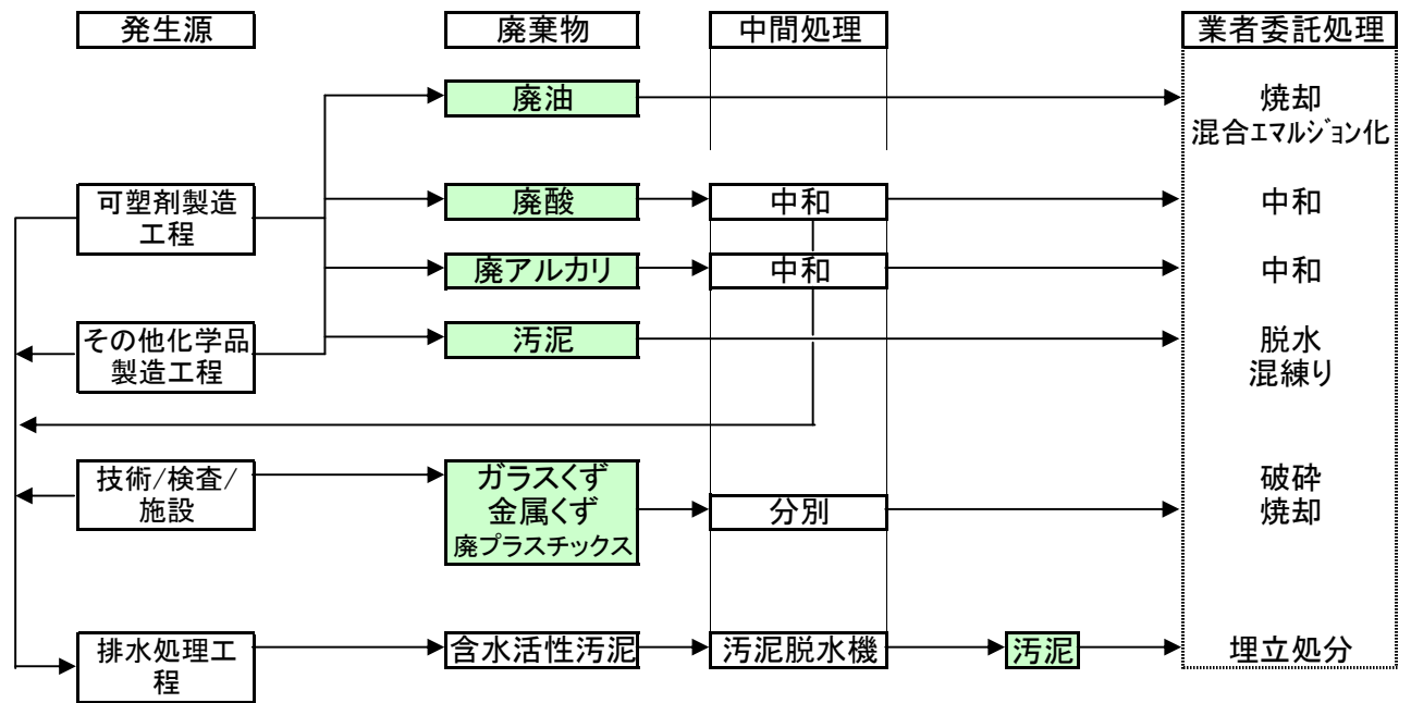
廃棄物処理フローシート(産業廃棄物)
