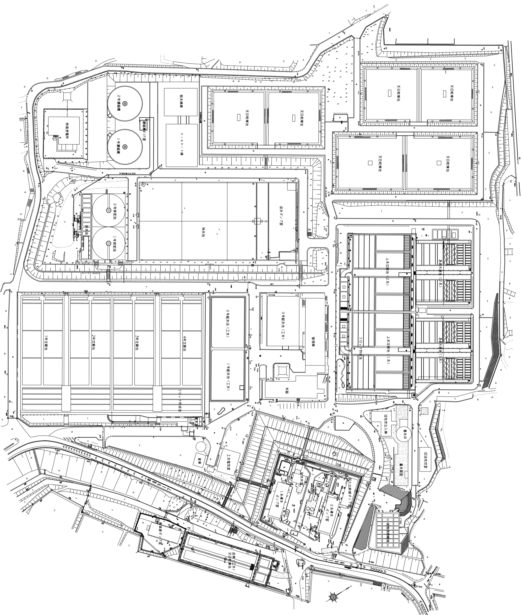
知多浄水場平面図
