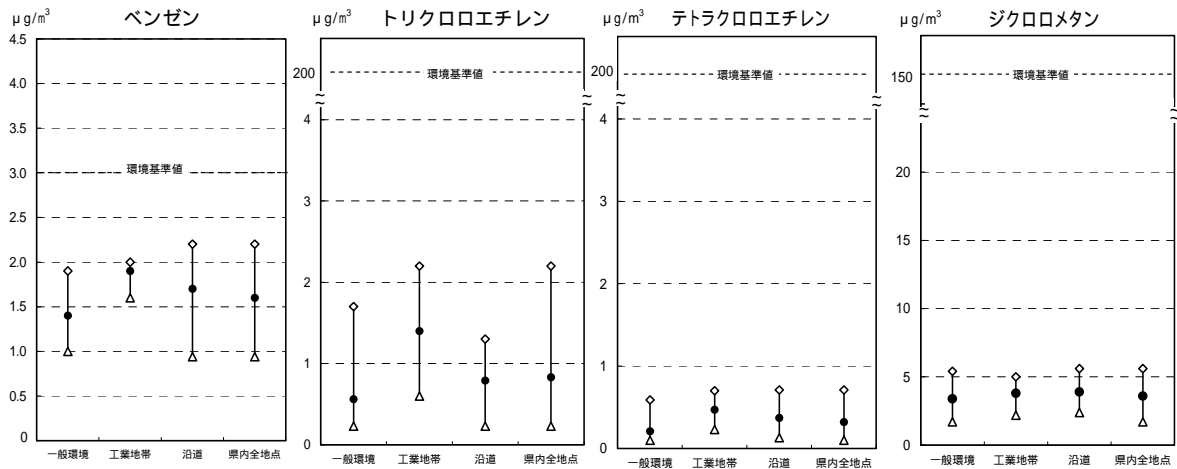
図 4 - 2 - 2 平成18年度における環境基準の定められている物質の調査結果 ( : 平均値 : 最大値 : 最小値 )
