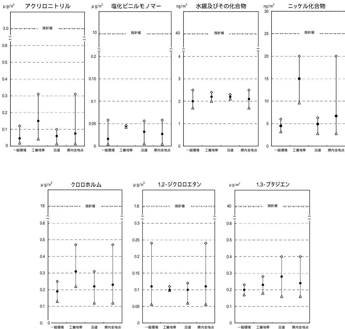
図 4 - 2 - 3 平成18年度における環境基準の定められている物質の調査結果
