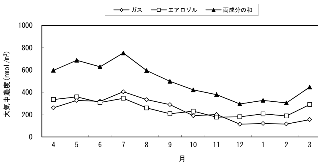
図6-11 ガス成分、エアロゾル成分大気中濃度の経月変化
