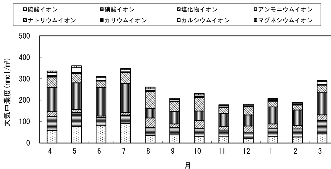
図6-10 エアロゾル成分の経月変化
