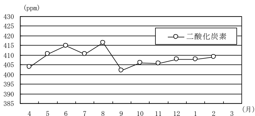
図 5－2 二酸化炭素の月平均値の推移
