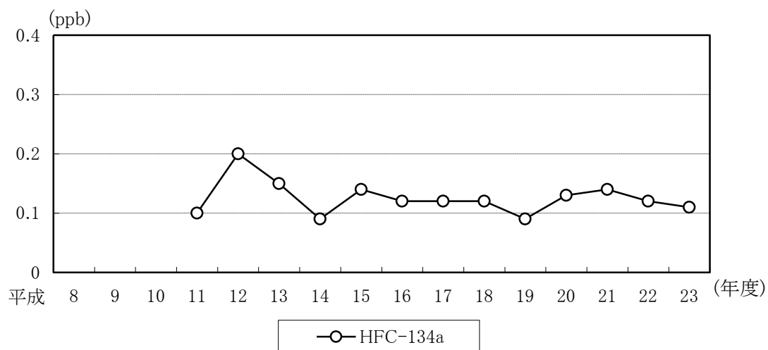
図 5－3 二酸化炭素等の年平均値の経年変化－（1）
