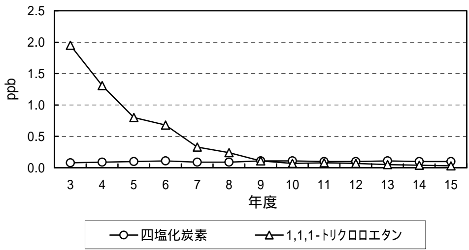
図5 - 3 二酸化炭素等の年平均値の経年変化 - ( 2 )
