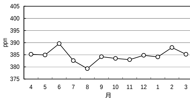
図 5 - 2 二酸化炭素の月平均値の推移
