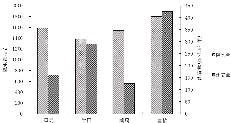
図 6-7 年間降水量と年間湿性沈着量の関係
