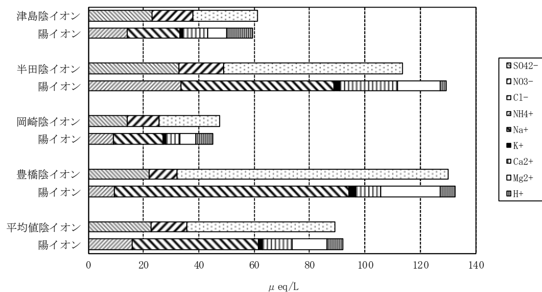
図6-5 イオン成分組成
