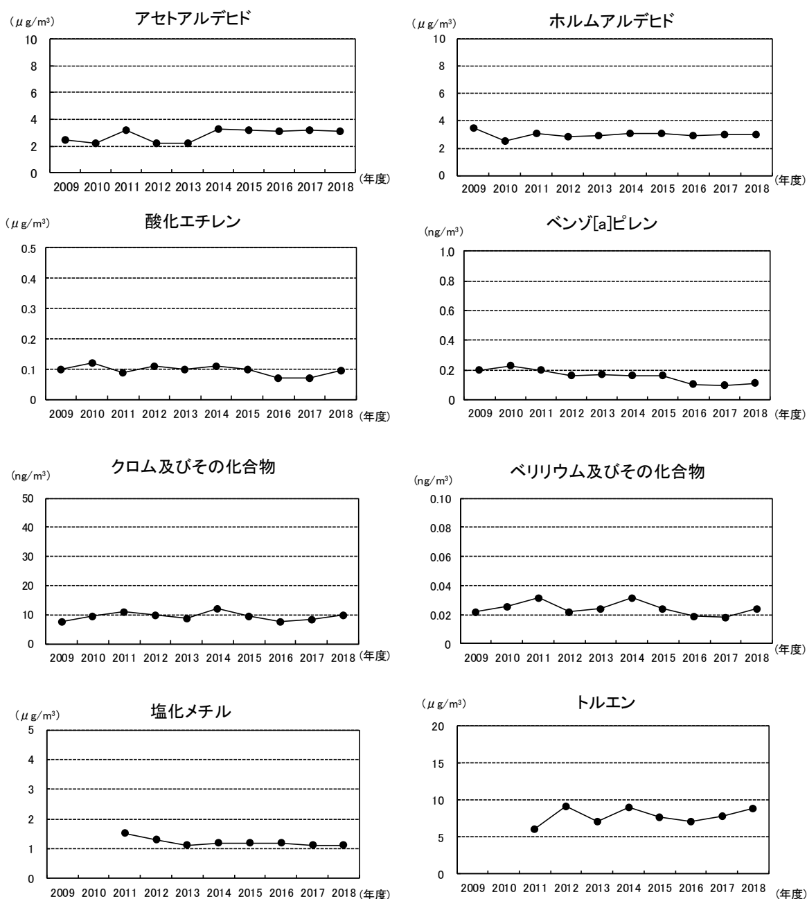
図 4 - 2 - 4 その他の物質の年平均値の経年変化
