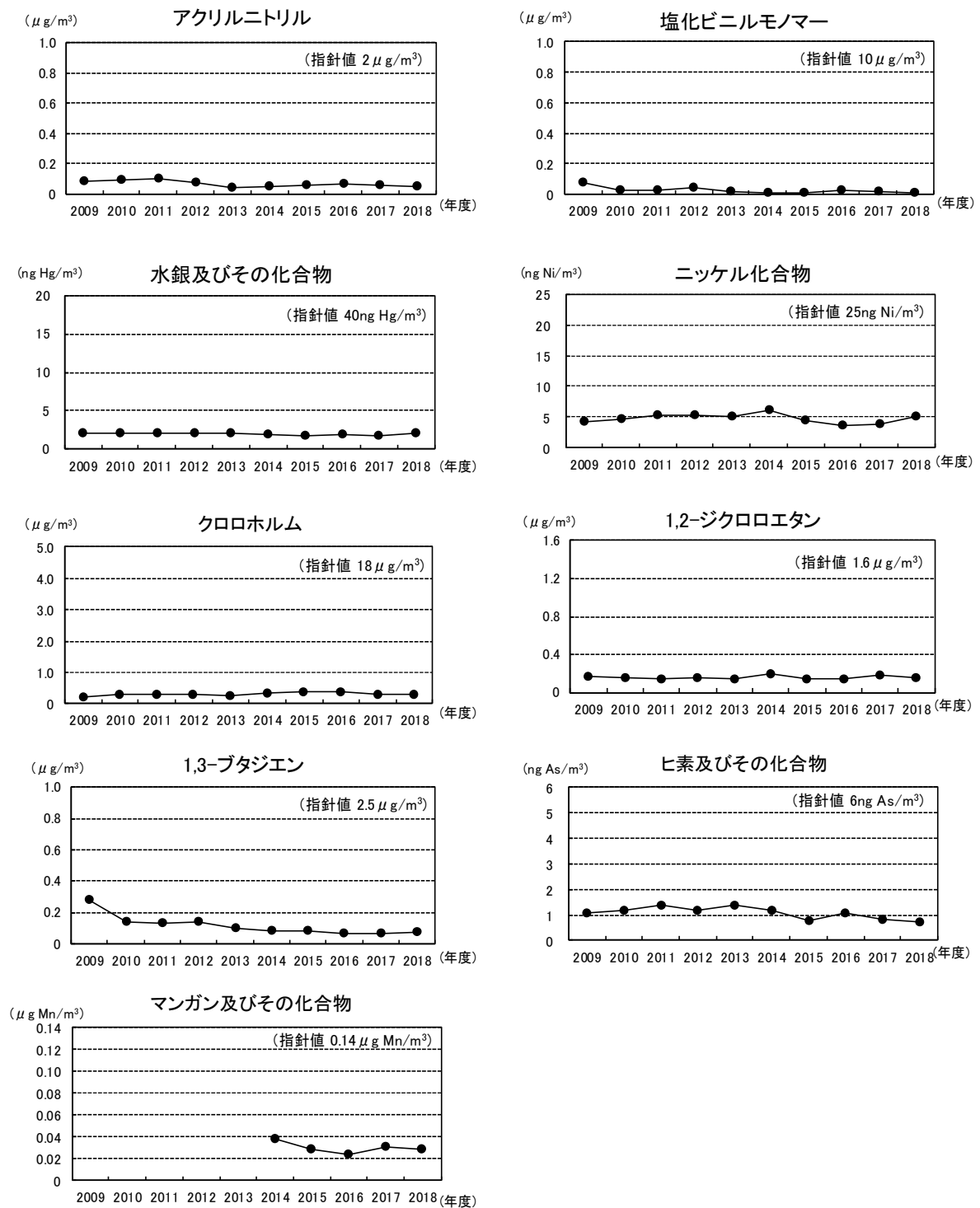
図 4-2-3 指針値の定められている物質の年平均値の経年変化
