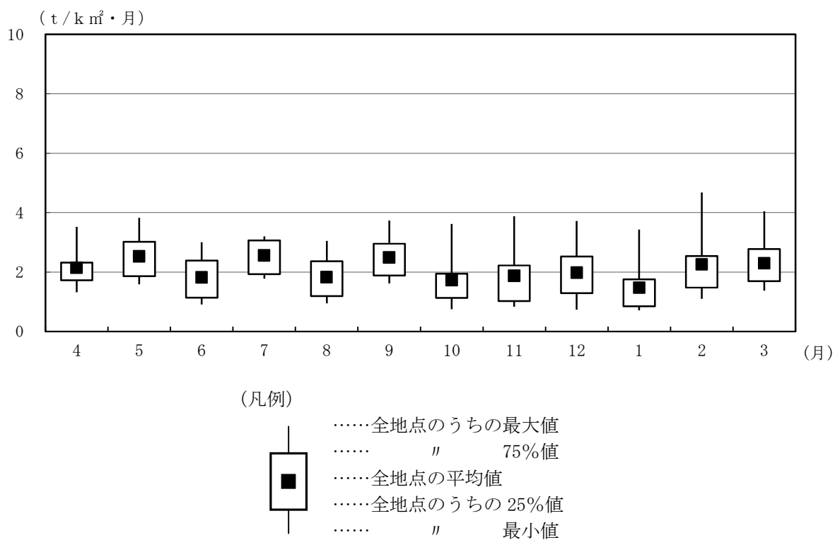
図8-2 降下ばいじん量（平成27年度）の経月変化
