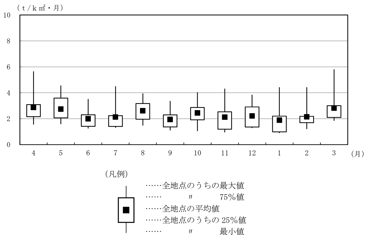
図8-2 降下ばいじん量(平成26年度)の経月変化
