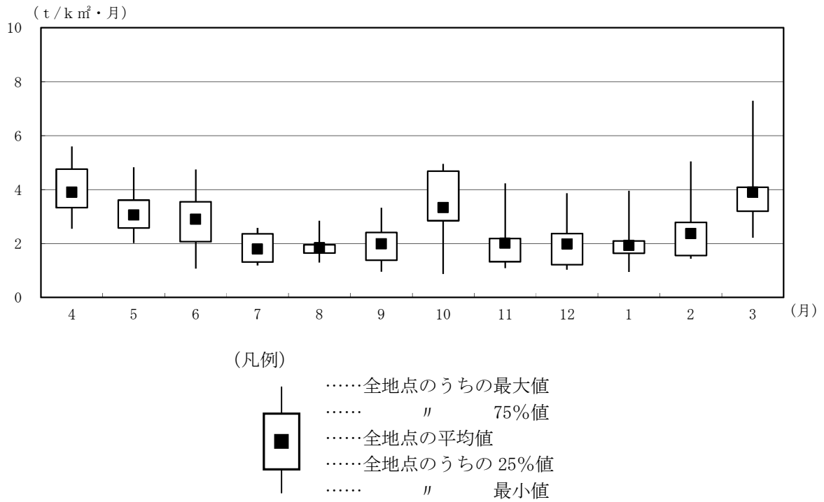
図8-2 降下ばいじん量（平成24年度）の経月変化
