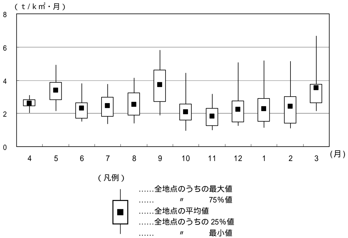
図8 - 2 降下ばいじん量 (平成 19 年度) の経月変化
