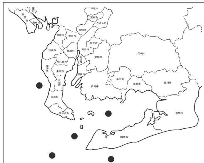
図 10-4-2 海水の採取地点
