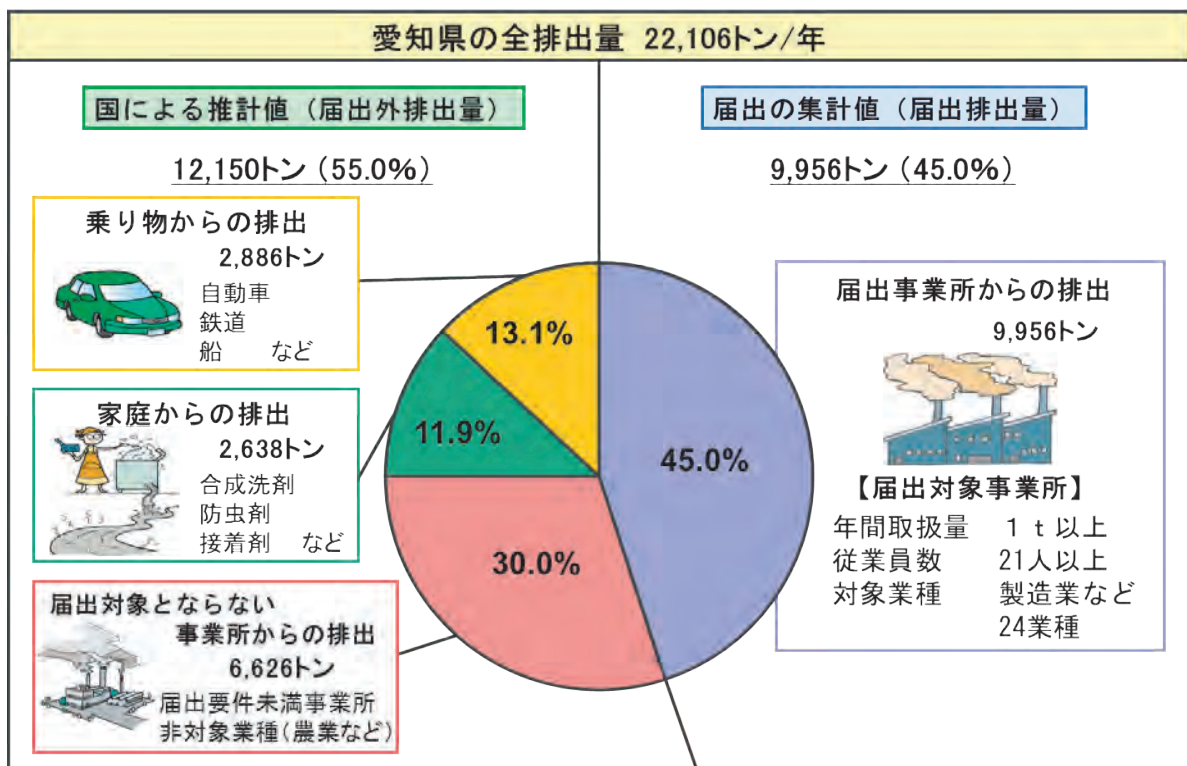
図10-1-3 排出量の排出源の内訳 (2018年度)
