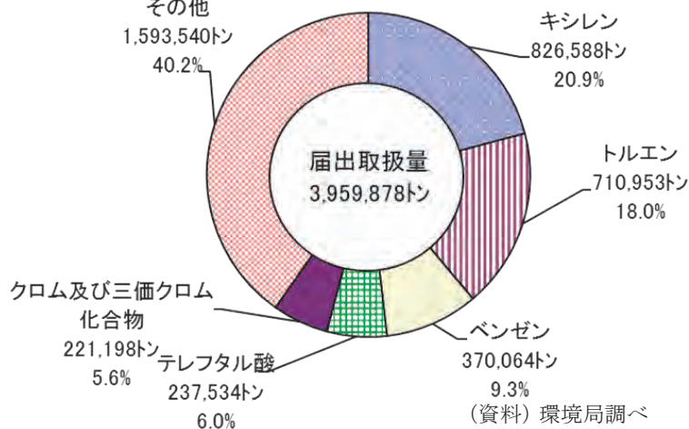
図 10-1-5 届出取扱量上位 5 物質とその割合 (2018 年度)
