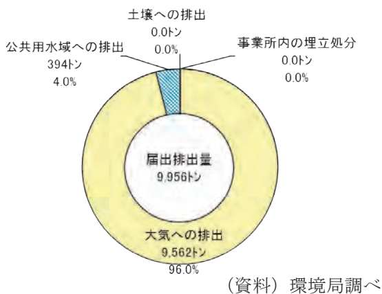
図10-1-1 届出排出量の排出先の内訳 (2018年度)
