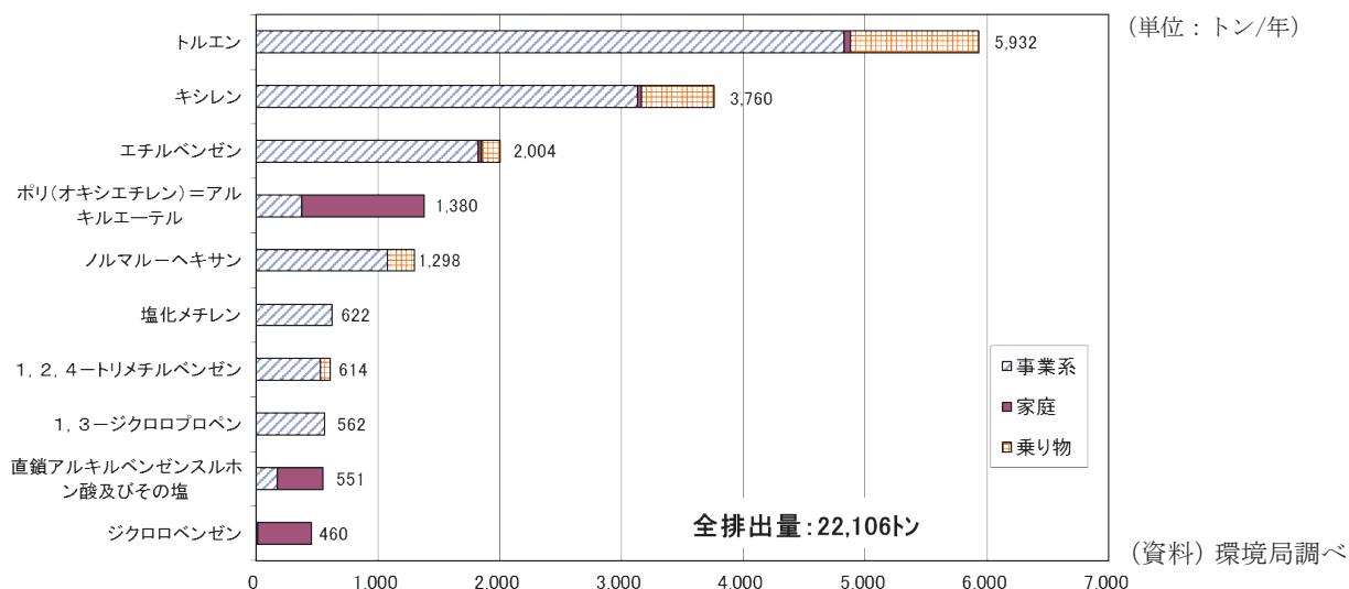
図 10-1-4 届出排出量・届出外排出量上位 10 物質とその発生源別排出量 (2018 年度)
