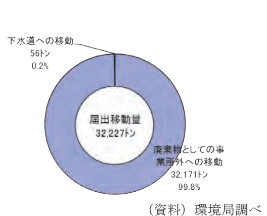
図10-1-2 届出移動量の移動先の内訳 (2018年度)
