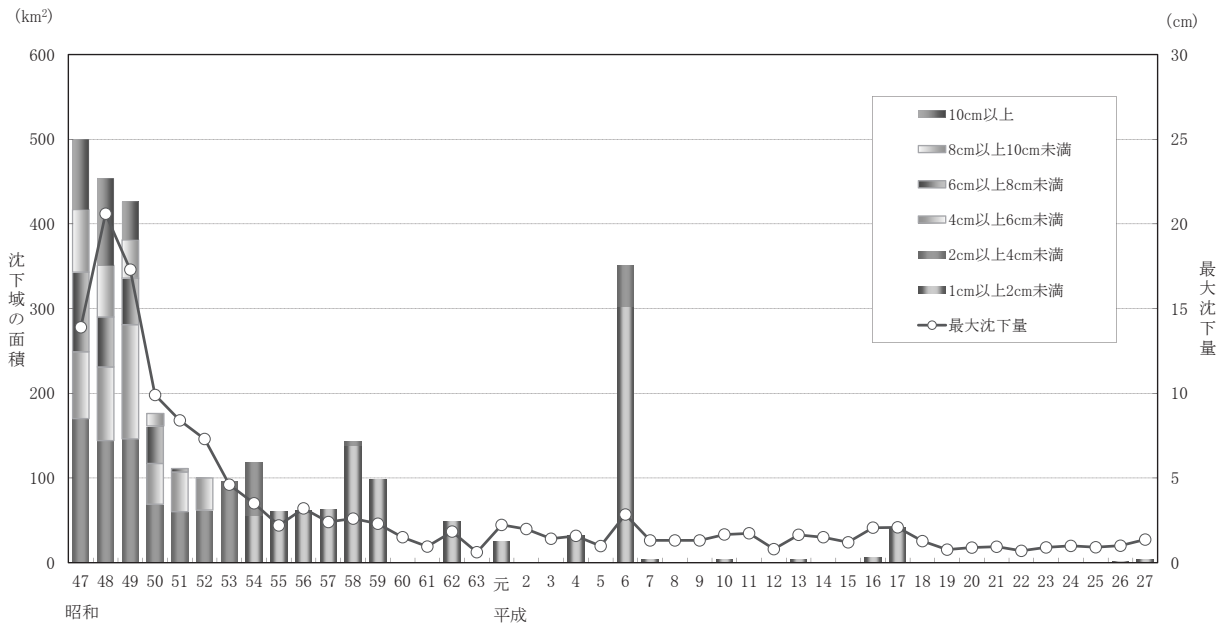
図1 沈下域及び最大沈下量の経年変化（尾張・名古屋市地域）
