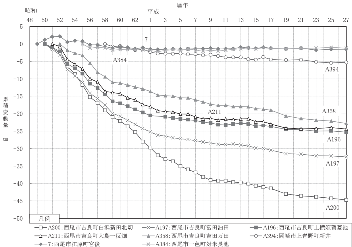
図4 主要な水準点の累積変動状況（西三河地域）
