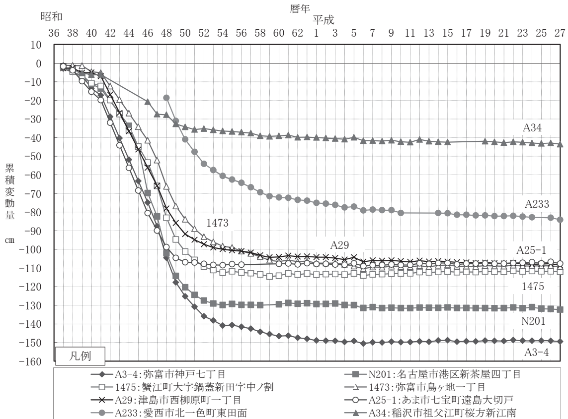
図3 主要な水準点の累積変動状況（尾張・名古屋市地域）
