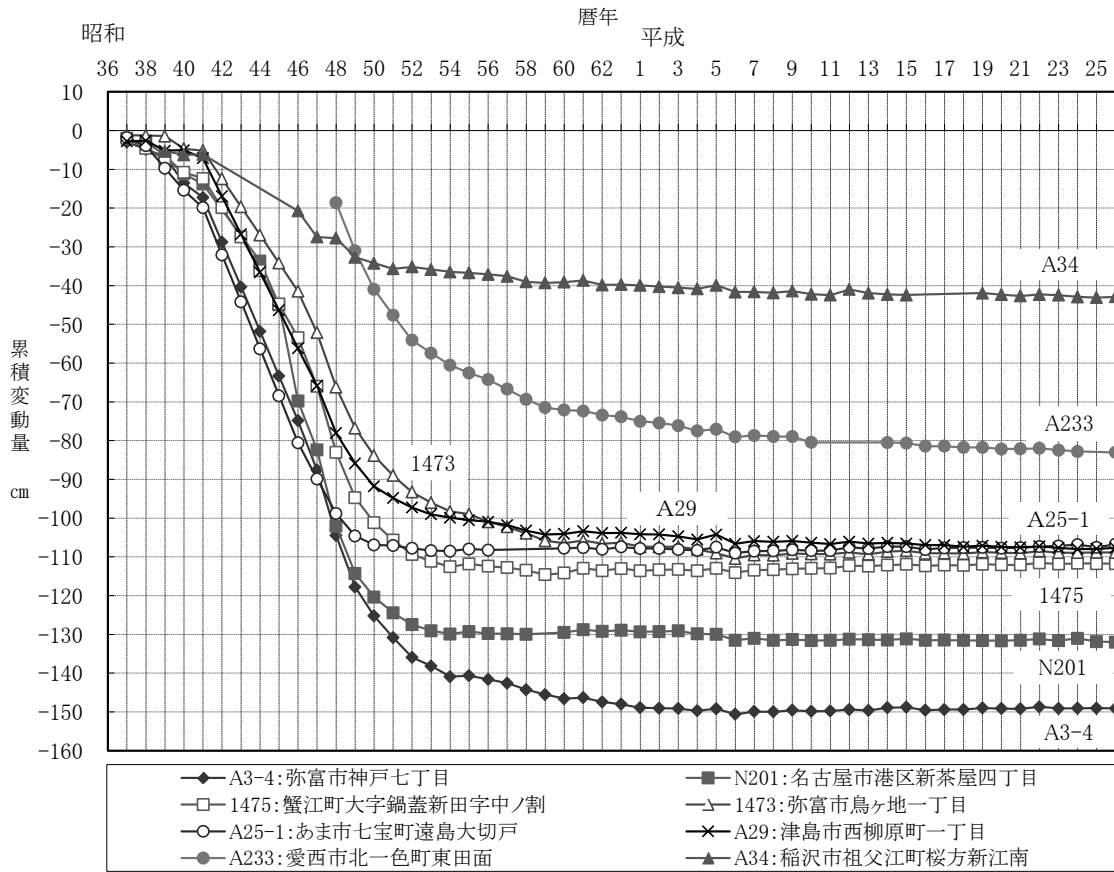
図3 主要な水準点の累積変動状況（尾張・名古屋市地域）
