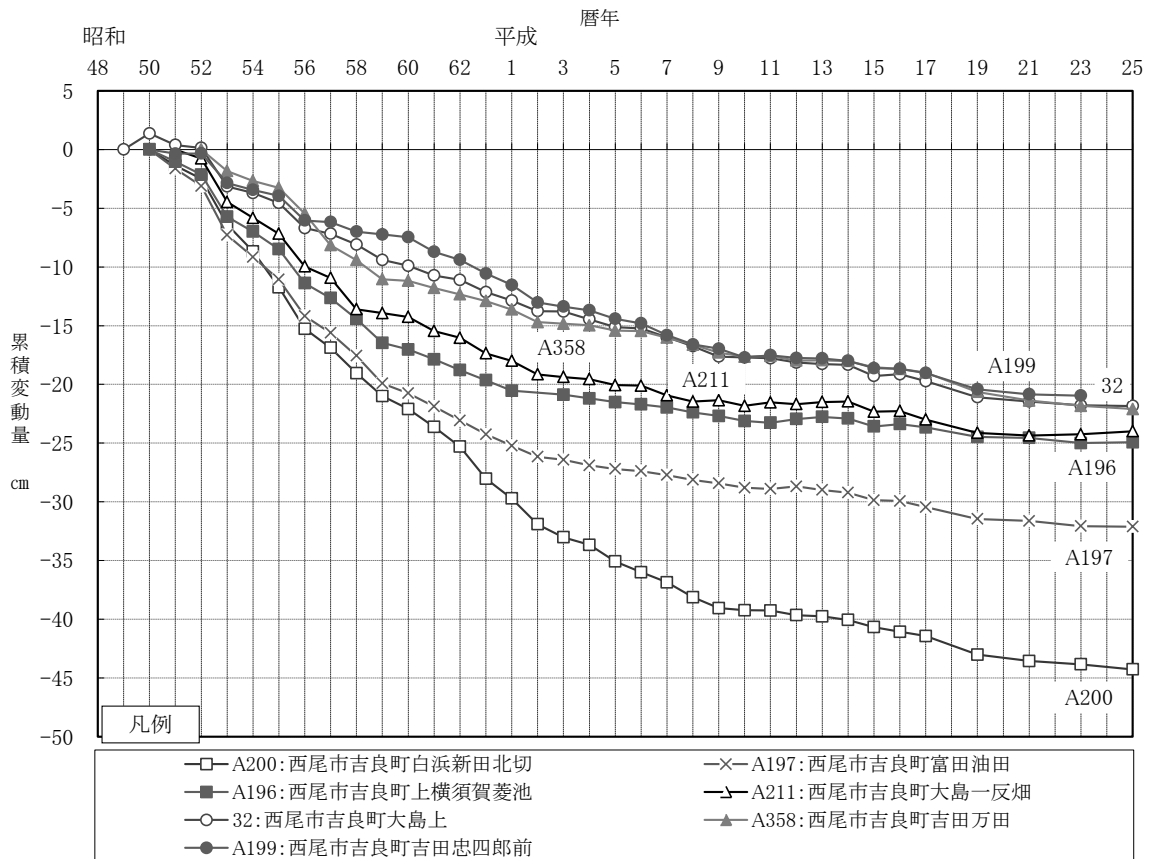
図4 主要な水準点の累積変動状況（西三河地域）
