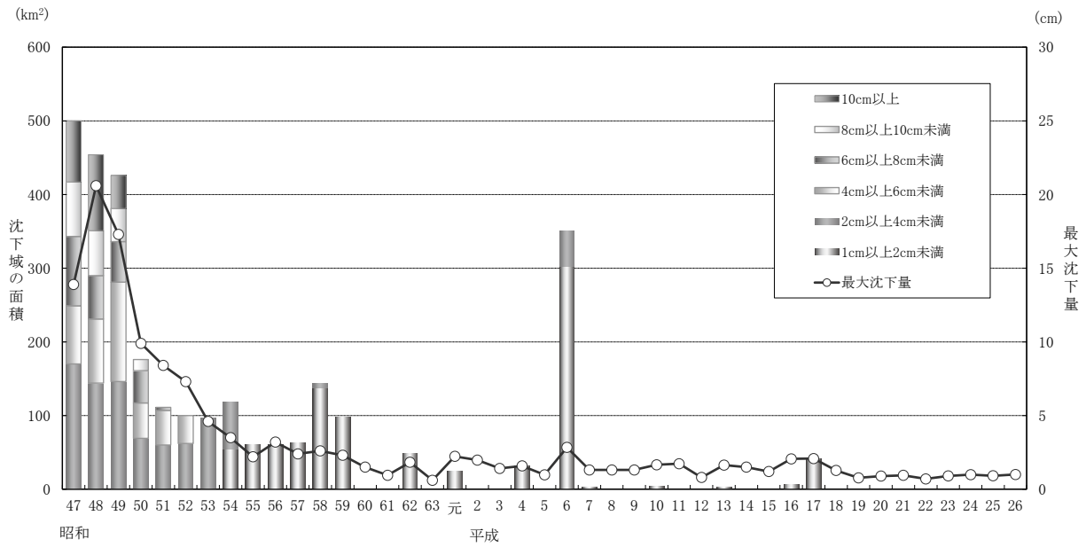
図1 沈下域及び最大沈下量の経年変化（尾張・名古屋市地域）
