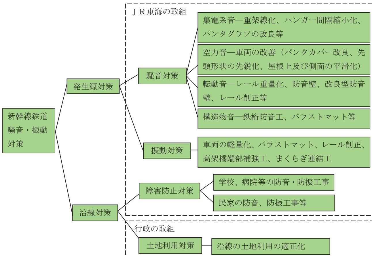
図 3-3-2 新幹線鉄道騒音・振動対策の体系
